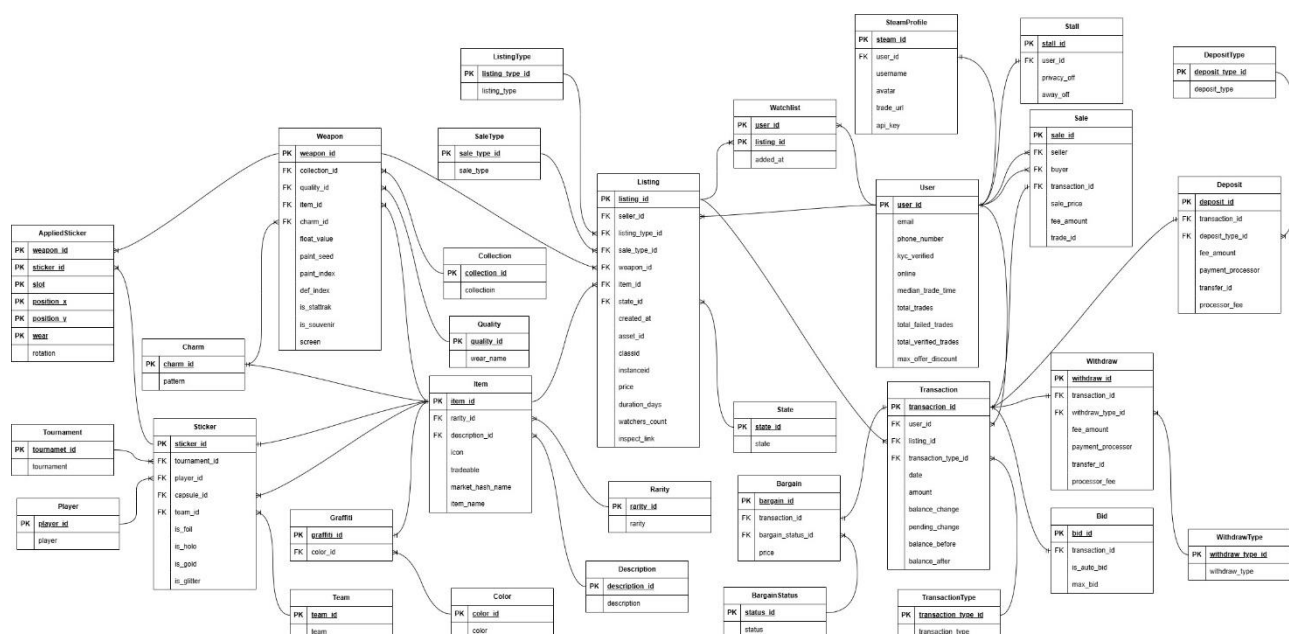
Рисунок 2.2.1 –ER-диаграмма проектируемой системы
